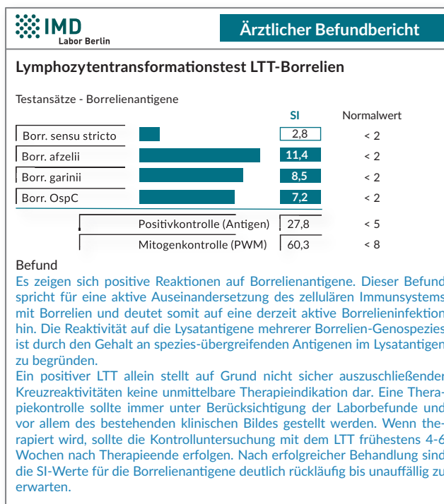
Abb. 1 Positiver LTT-Musterbefund
